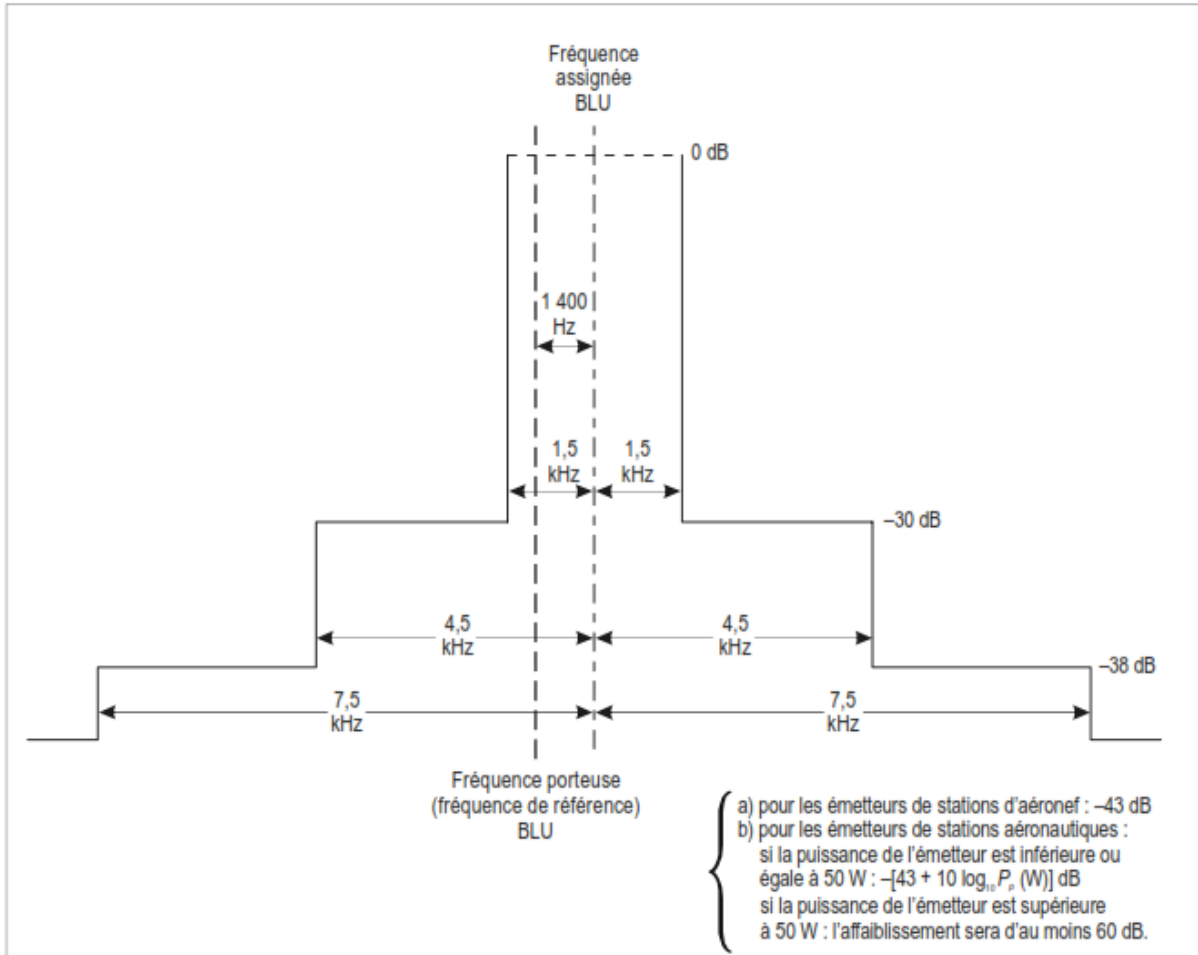
Figure 2-2. Limites du spectre requises (sous forme de puissance de crête) pour les émetteurs de stations d'aéronef installés pour la première fois après le 1 er février 1983 et pour les émetteurs de stations aéronautiques en service après le 1 er février 1983
