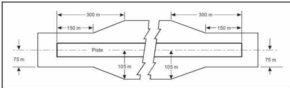
Figure A-4. Partie nivelée d'une bande de piste avec approche de précision lorsque le chiffre de code est 3 ou 4
