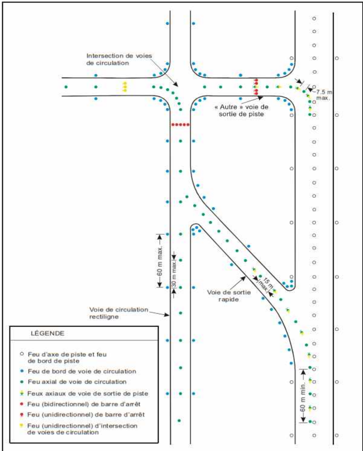
FIGURE 5-26 BALISAGE LUMINEUX DE VOIE DE CIRCULATION
