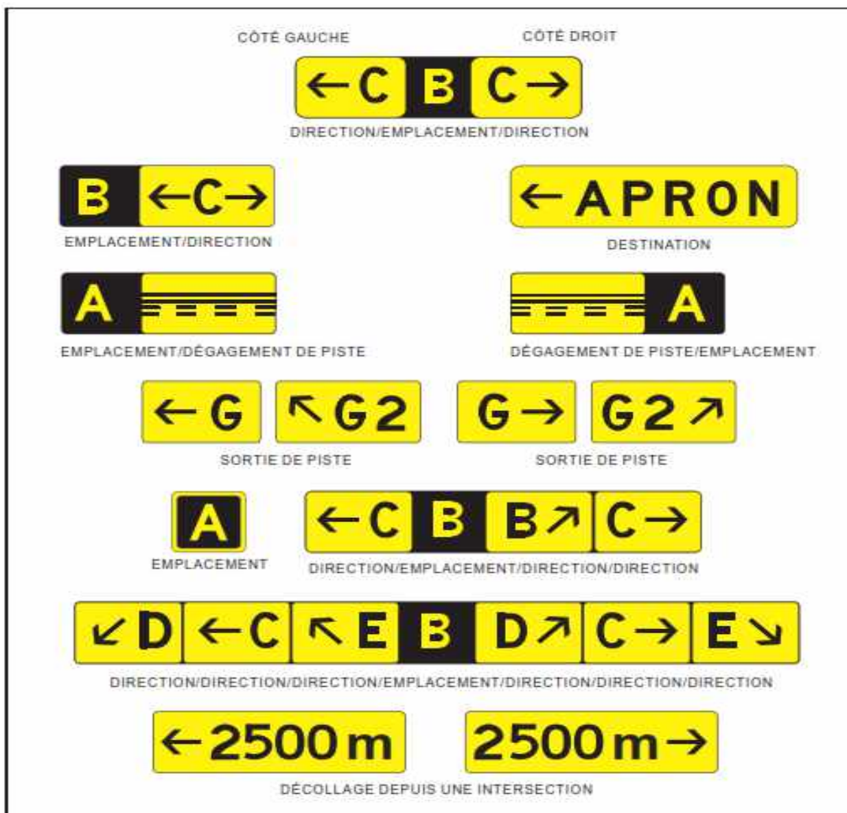
Figure 5-31. Panneaux d'indication
