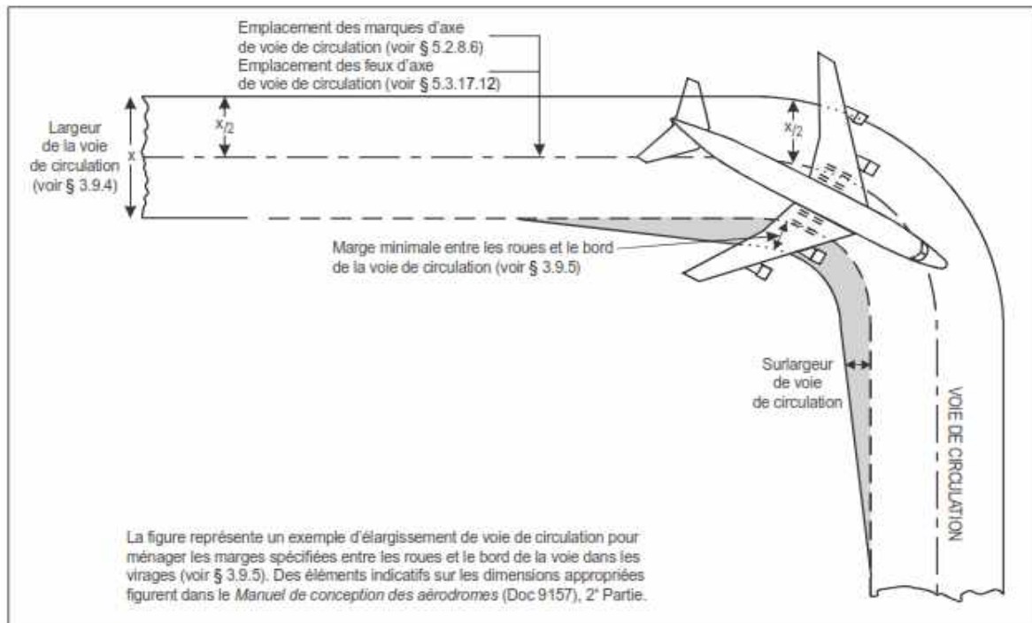
Figure 3-2. Virage de voie de circulation
