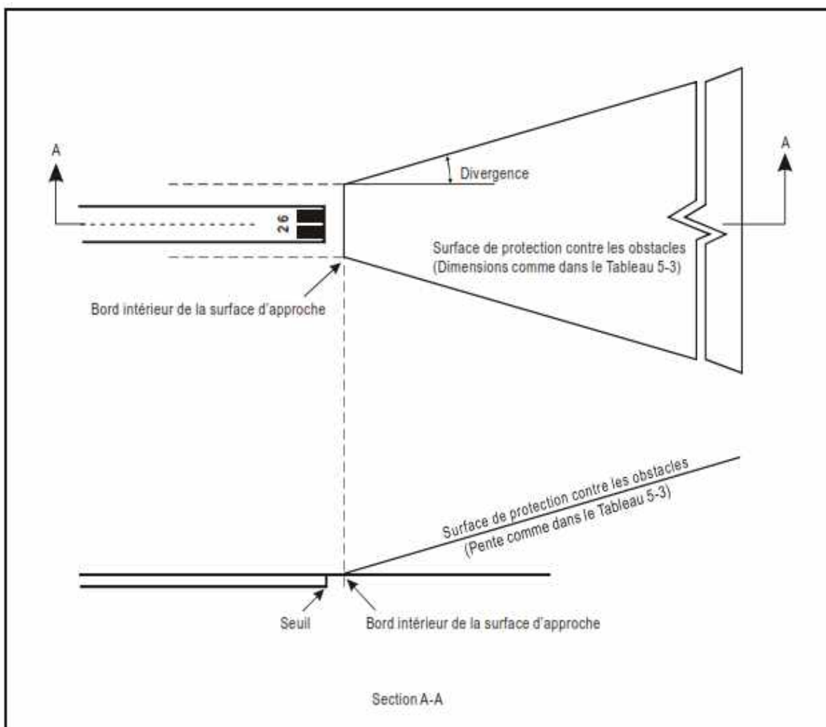
Figure 5-21. Surface de protection contre les obstacles pour les indicateurs visuels de pente d'approche
