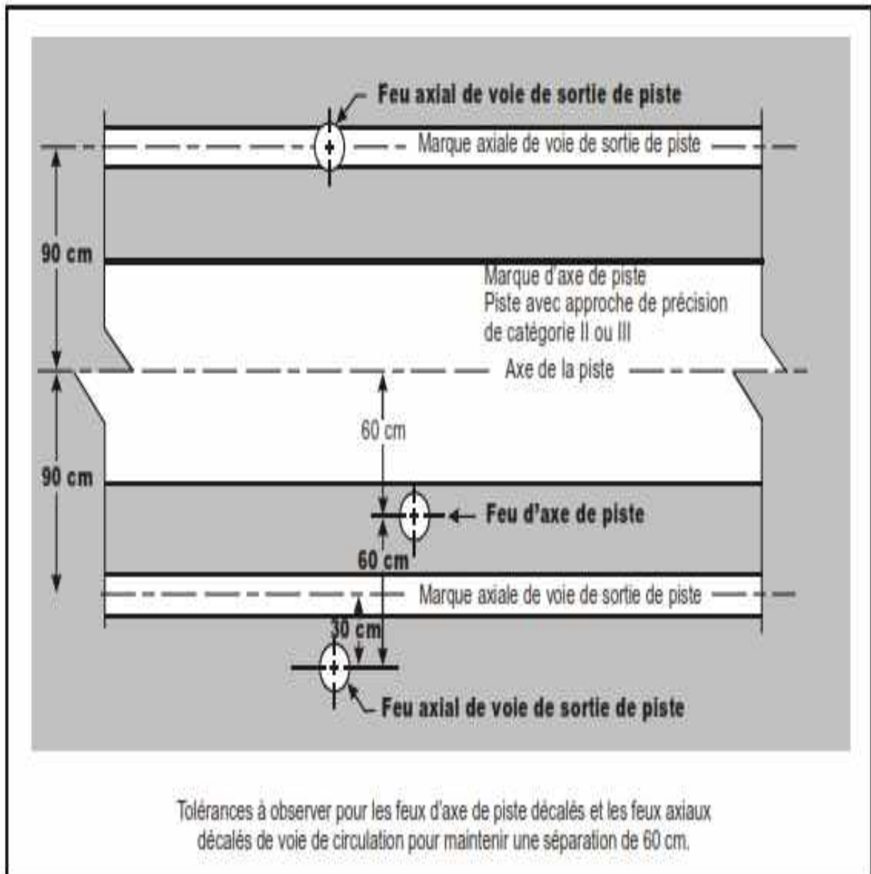
Figure 5-27. Feux d'axe de piste décalés et feux axiaux décalés de voie de circulation
