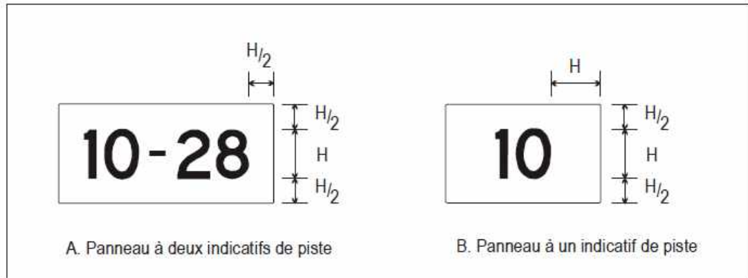
Figure A4-4. Dimensions des panneaux
