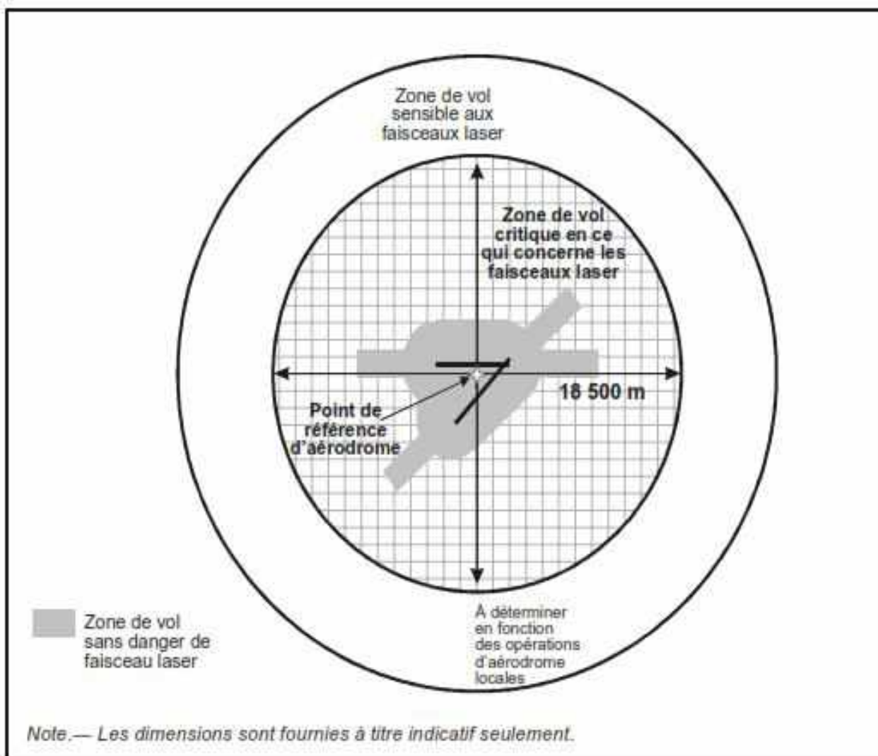
Figure 5-11. Zones de vol protégées
