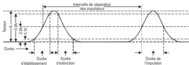
Figure 3-1. Définitions des formes d'onde du radar secondaire de surveillance, des intervalles de temps et du point de référence de sensibilité et de puissance du transpondeur.
