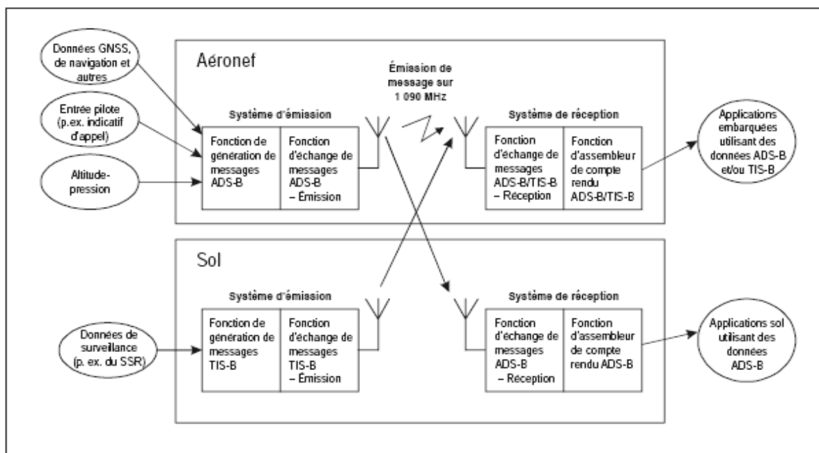
Figure 5-1. Modèle fonctionnel de système ADS-B/TIS-B
