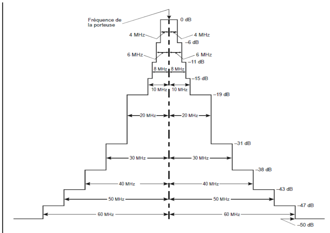
Figure 3-2. Limites du spectre pour l'interrogateur
